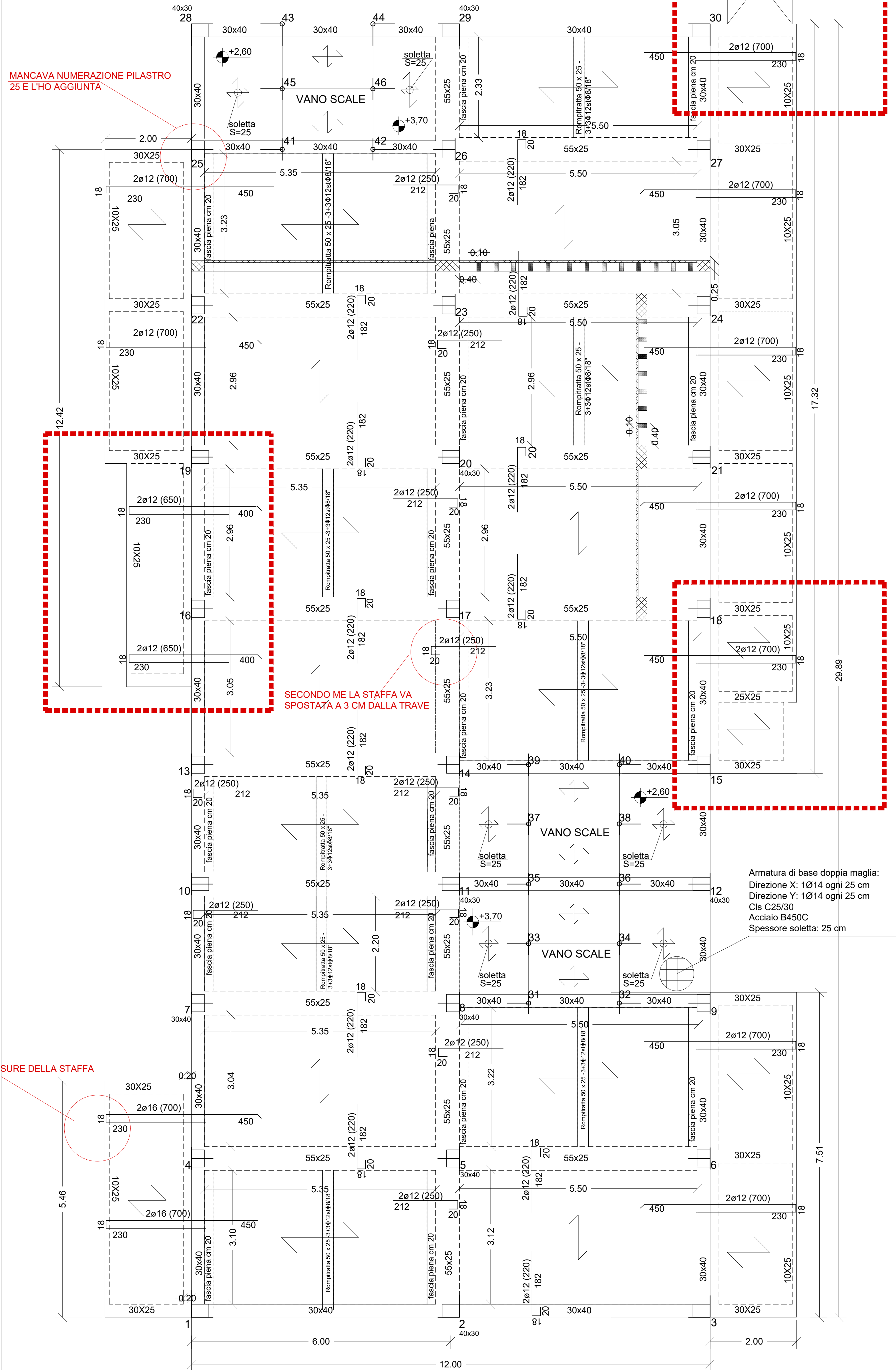
Pianta al livello 2 - Quota 3.70 m
